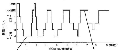
一晩の眠りの深さや種類を表した図
