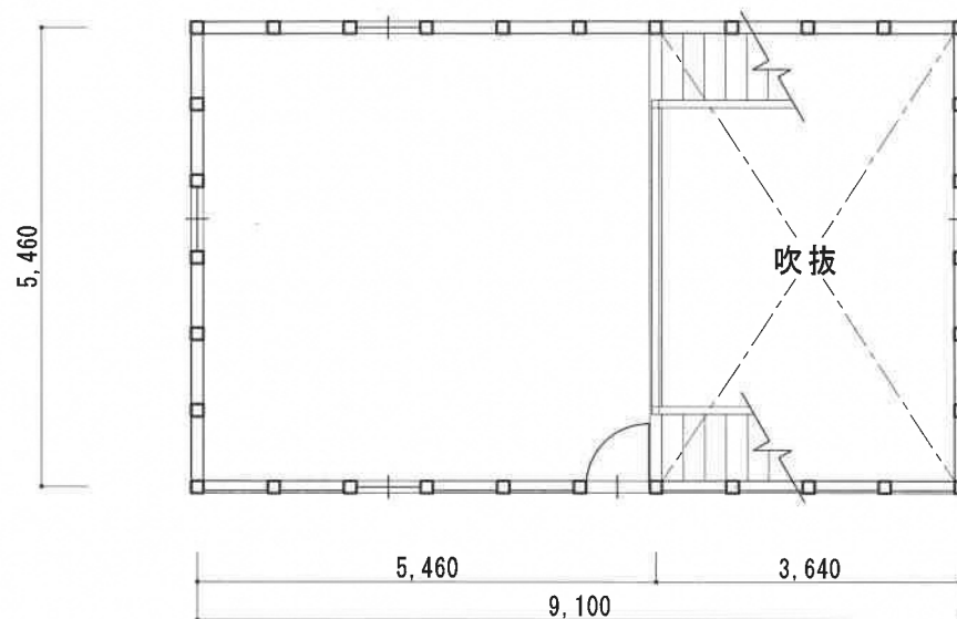
2F平面図 1/100
