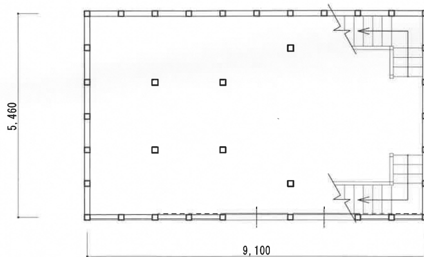
1F平面図 1/100
